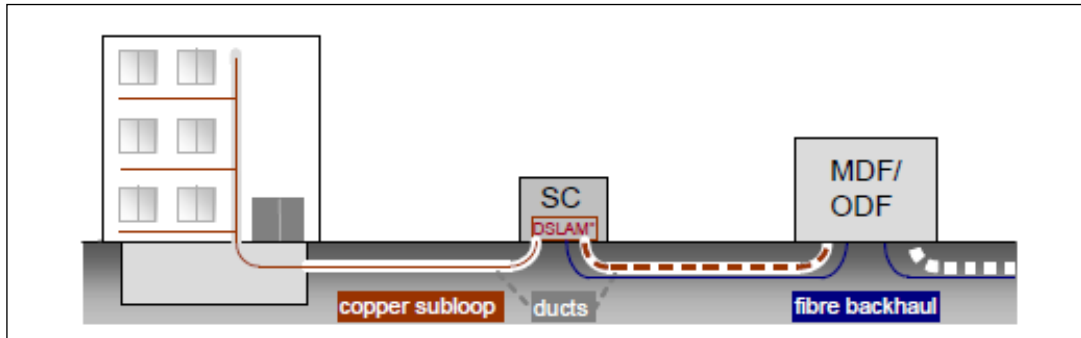
Slika 5: FttCab rješenje
