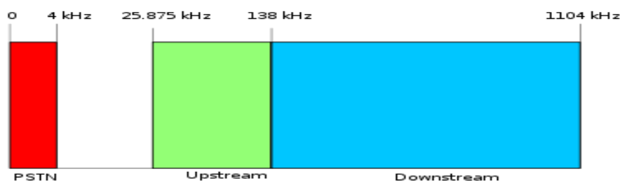
Slika 2. Podjela frekvencijskog opsega kod ADSL tehnologije
