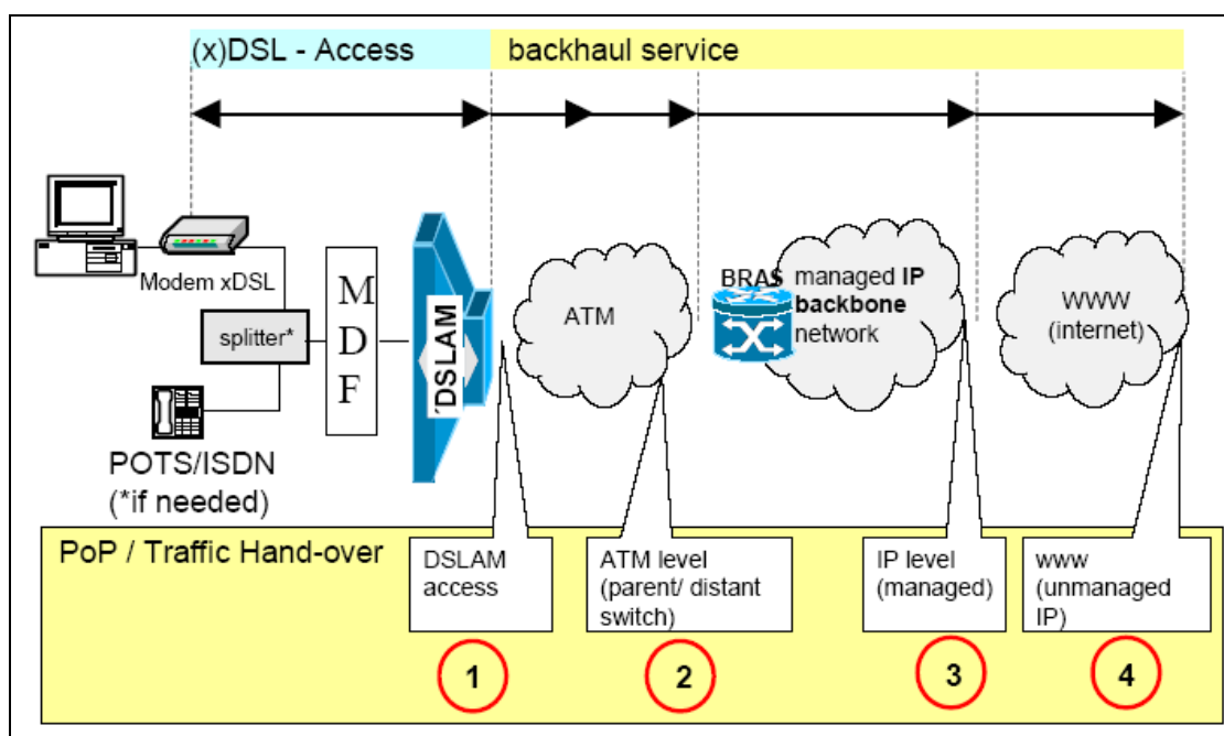
Slika 4. Tačke preuzimanja DSL saobraćaja
