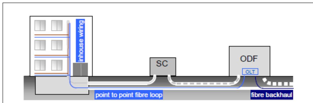
Slika 6: FttH rješenje (point-to-point)
