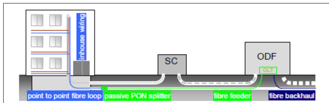
Slika 7: PON arhitektura (point-to-multipoint)
